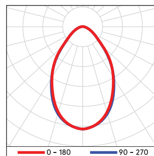
Linear Module
